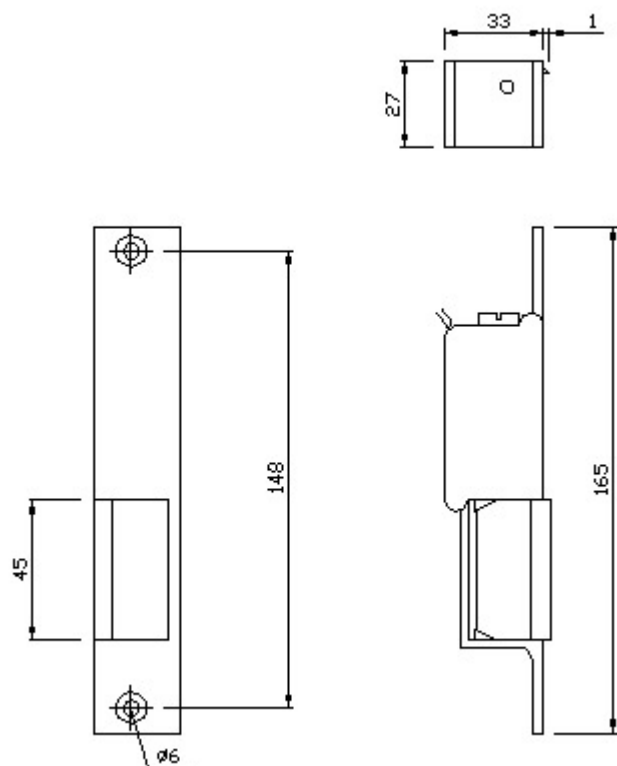
Wymiary i zdjęcie zaczeu
